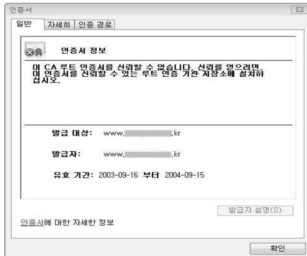
〈그림 3-10〉 인증서 오류 원인 확인 방법
