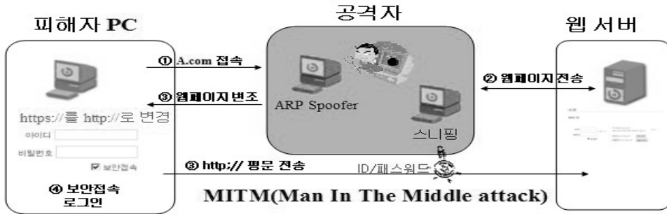
〈그림 D-2〉 ARP 스푸핑과 데이터 변조를 통한 MITM 공격
