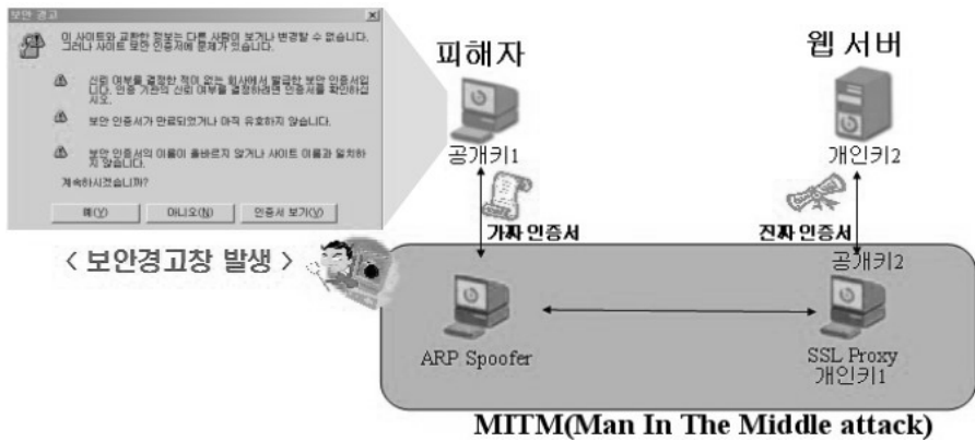
<그림 D-1> ARP 스푸핑을 이용한 MITM 공격
