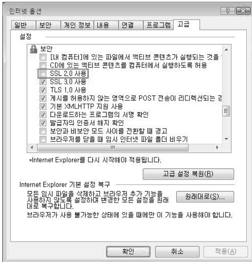
〈그림 3-11〉 IE 7의 인증서 프로토콜 기본 설정
