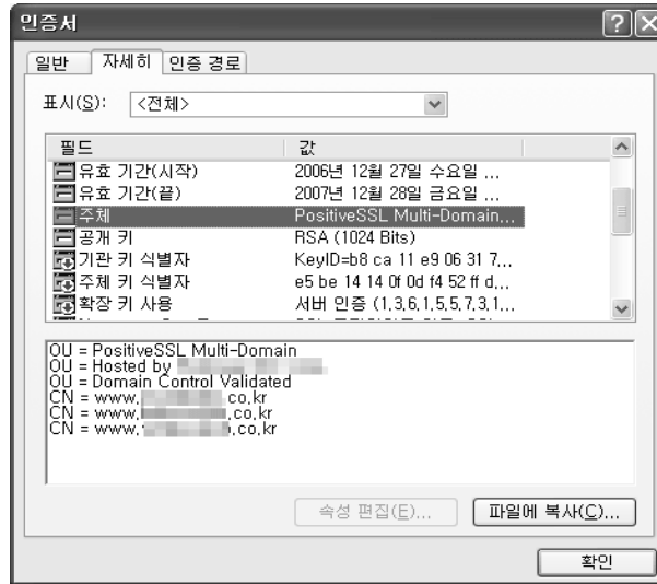
〈그림 B-3〉 다수의 CN이 포함된 멀티도메인 SSL 인증서
